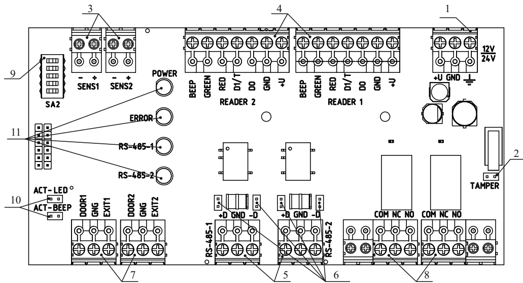
Рисунок 4 – Плата модуля
