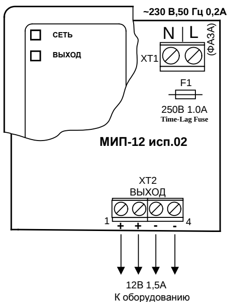
Рис. 3 Схема подключения МИП-12 исп.02 (МИП-12-1/ПЗ)
