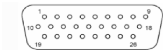
Рисунок 2 – Распиновка разъема на передней панели
