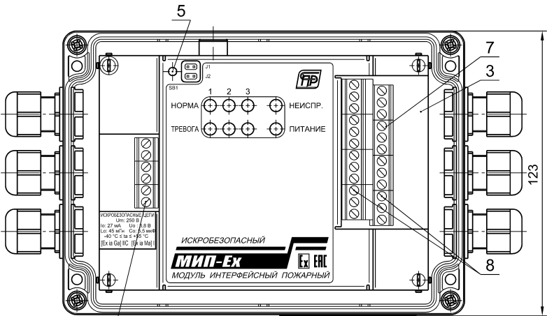
МИП-3И-Ех
