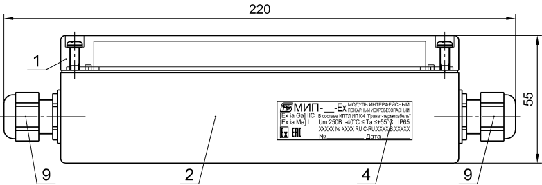
МИП-3-Ех
