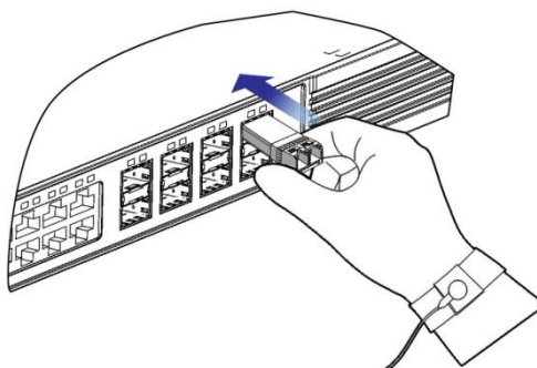
Рисунок 5-18. Установка SFP/SFP+-модулей
