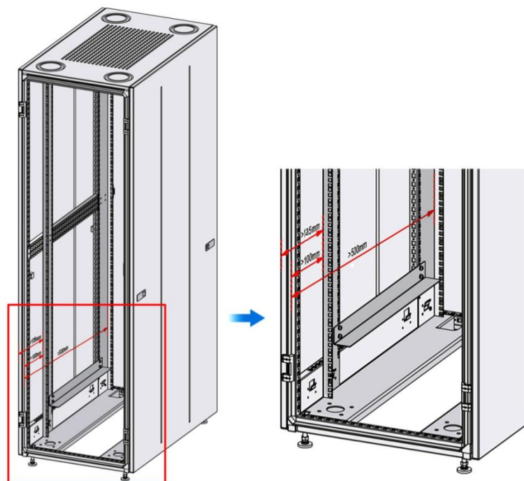
Рисунок 4-2. Размеры шкафа
