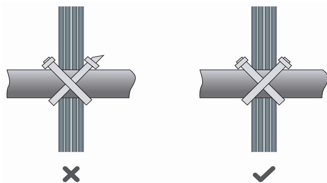
Рисунок 13-2. Правильная обрезка стяжки для кабелей
