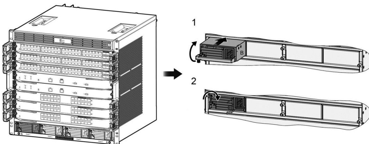
Рисунок 5-9. Установка модуля питания
