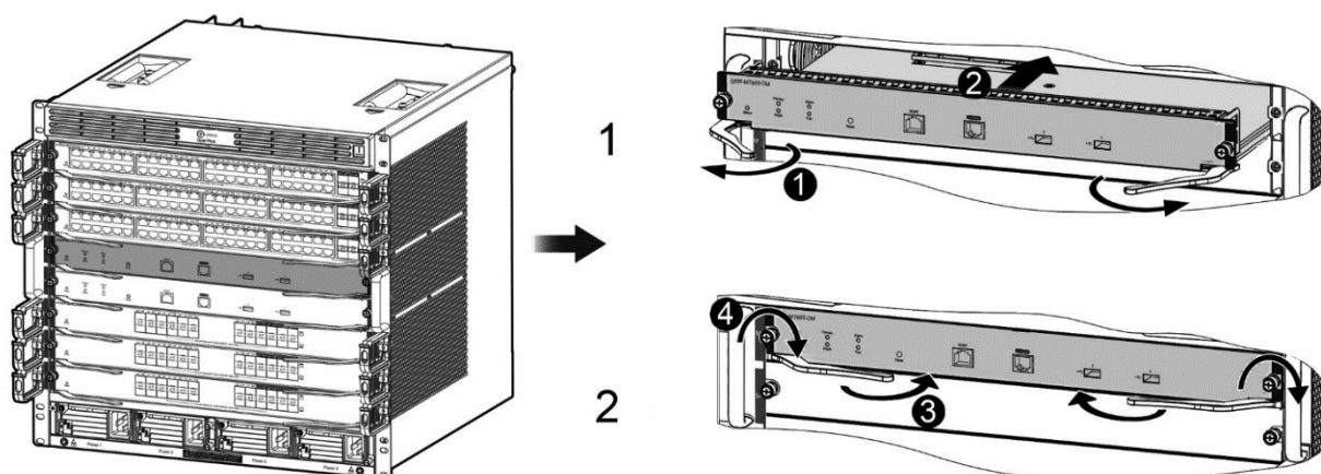
Рисунок 5-15. Установка модулей в QSW-7608
