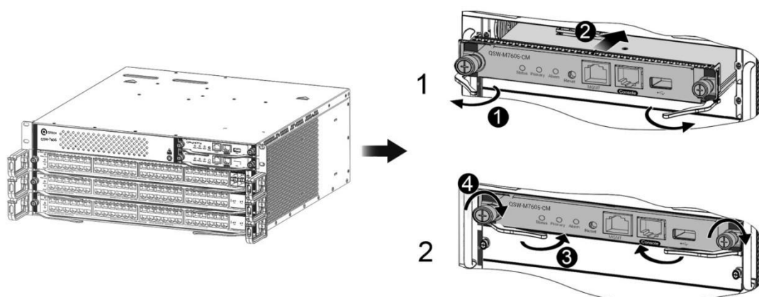
Рисунок 5-16. Установка модулей в QSW-7605
