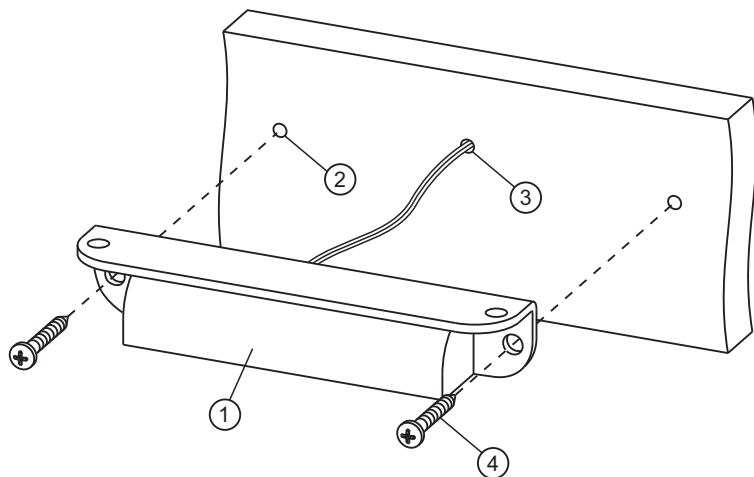
Крепление модуля на вертикальную металлическую поверхность с использованием винтов самосверлящих
