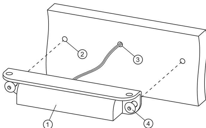
Крепление модуля на вертикальную металлическую поверхность с использованием заклёпок
