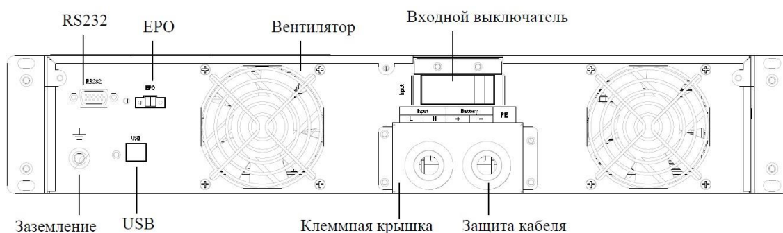
Рисунок 2-2. Задняя панель
