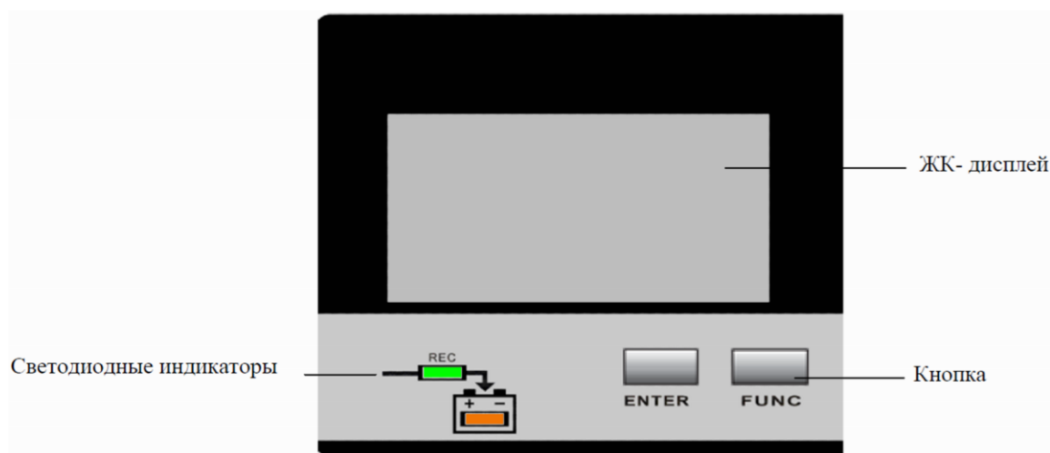
Рисунок 4-1. Панель управления
