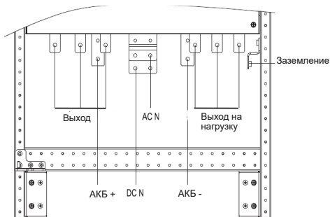
Рисунок 14 – Шина с клеммами системного шасси ИБП 125 кВА со стороны передней панели
