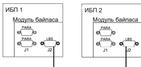
Рисунок 37– Подключение LBS портов
