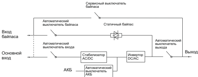
Рисунок 10 – Структура ИБП
