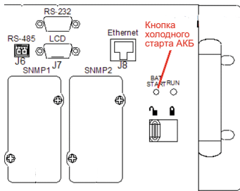
Рисунок 32 – Кнопка холодного старта АКБ
