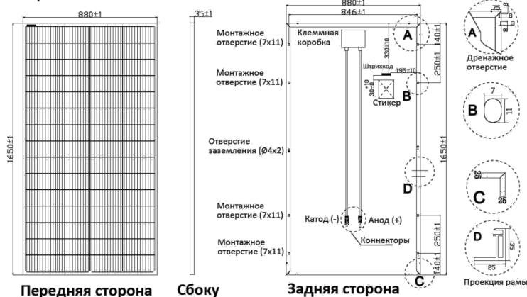
Габариты: мм
