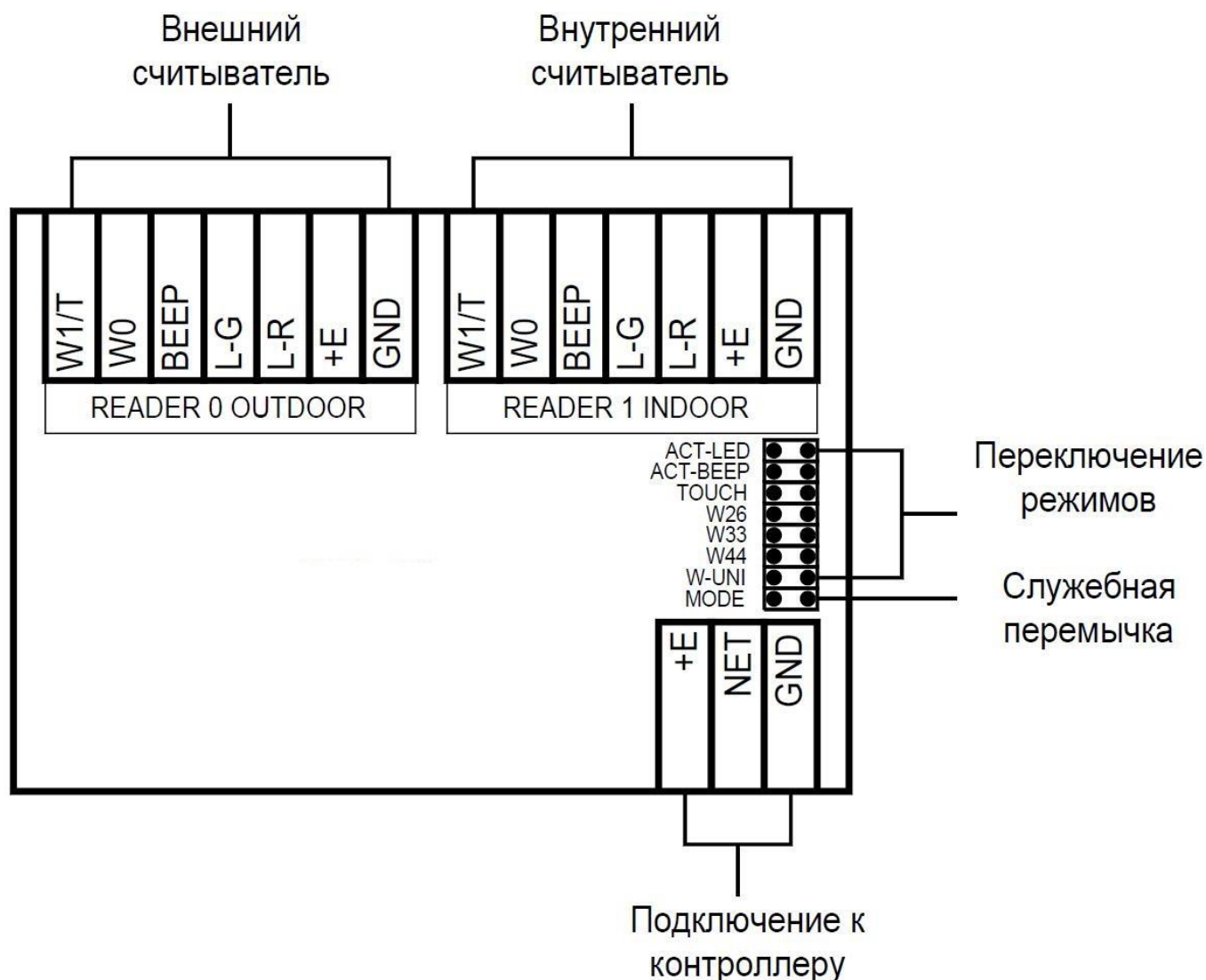
Рисунок 2. Схема платы интерфейса ЛКД-МКС-02
