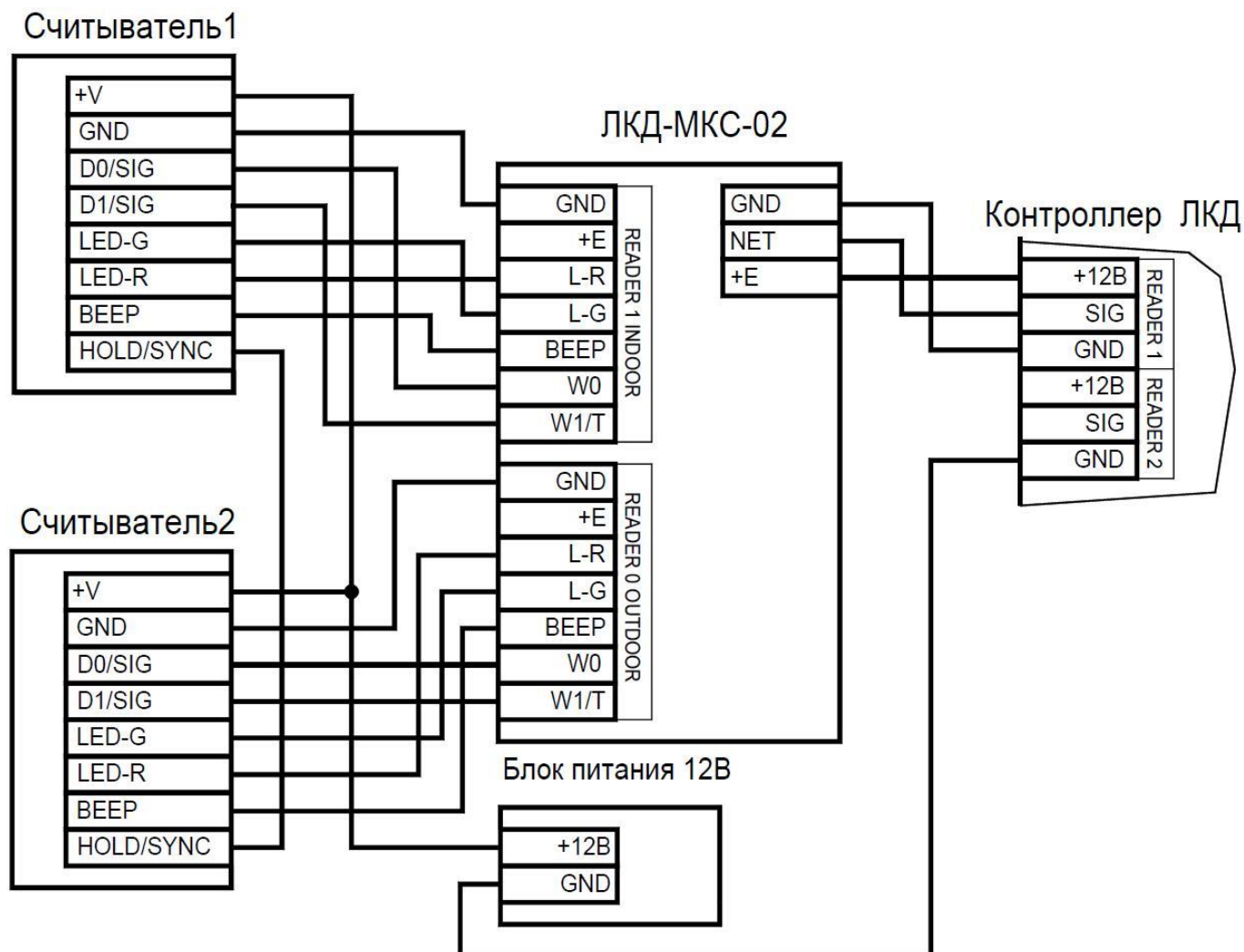
Рисунок 5. Подключение считывателей с питанием от внешнего источника
