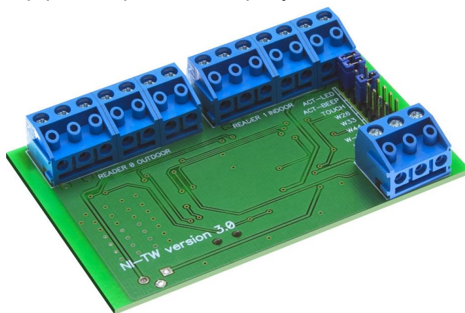
Рисунок 1. Интерфейс сопряжения ЛКД-МКС-02
