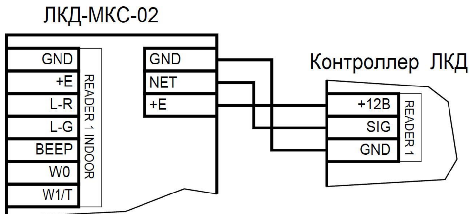
Рисунок 4. Подключение интерфейса ЛКД-МКС-02 к контроллеру
