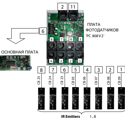
Модуль приемника
