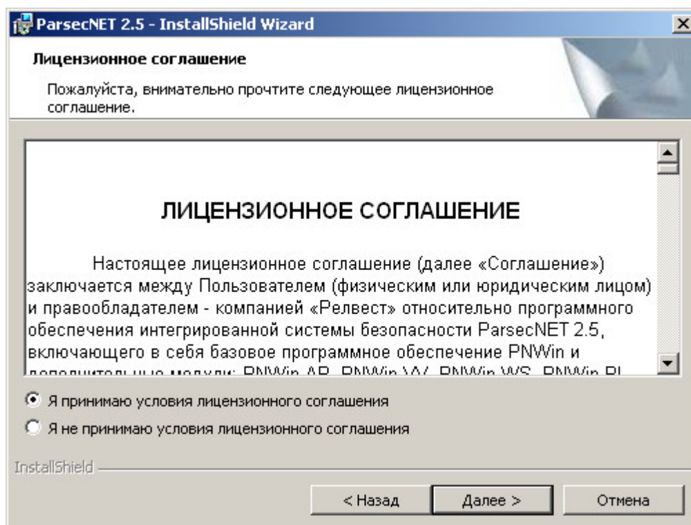
Лицензия
