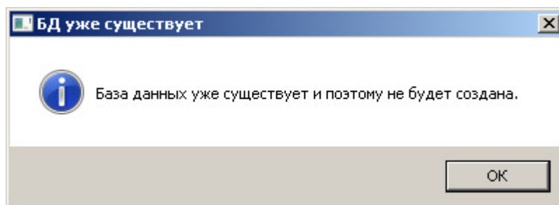
Системное сообщение
