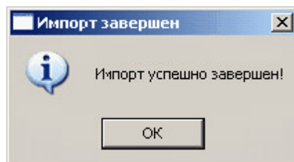
Системное сообщение
