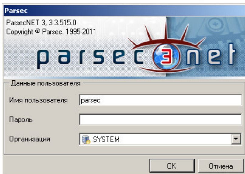
Авторизация ParsecNET 3
