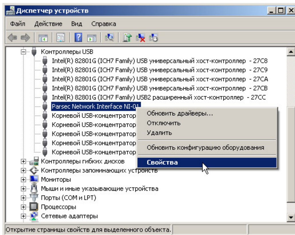
Диспетчер устройств
