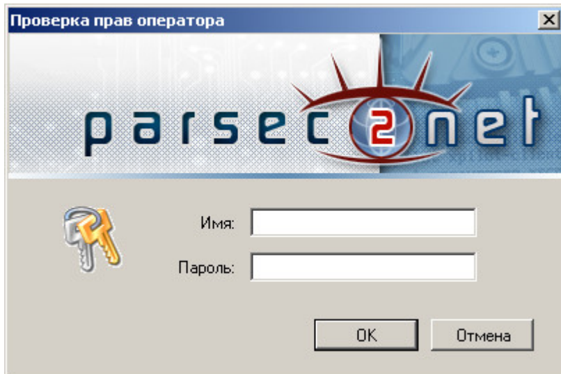
Авторизация ParsecNET 2.5
