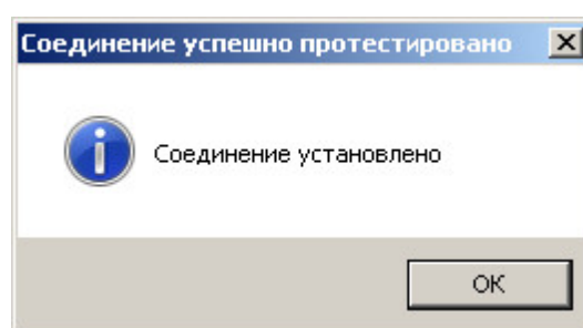
Системное сообщение
