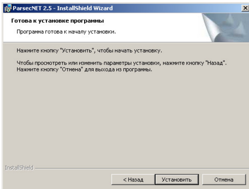
Ход установки
