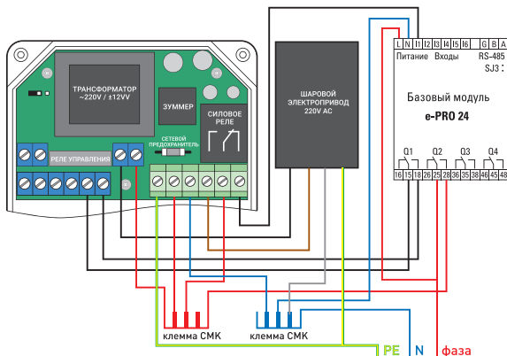
Рис. 8 Схема подключения
