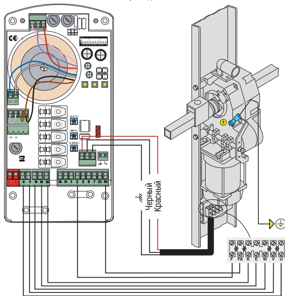
Привод E306/E456
