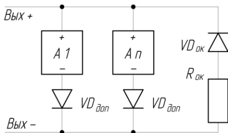
Рисунок 2 – Схема подключения ШС УС
