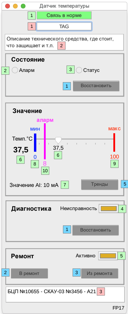
Рис. 17 Внешний вид FP17
