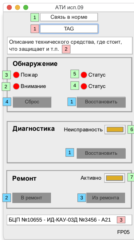
Рис. 5 Внешний вид FP05
