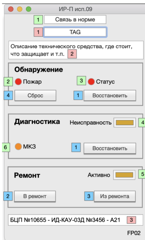
Рис. 2 Внешний вид FP02
