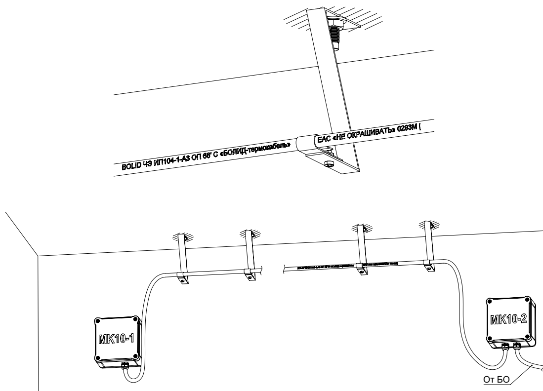
Рисунок 2. Пример размещения МЭТ-01-01
