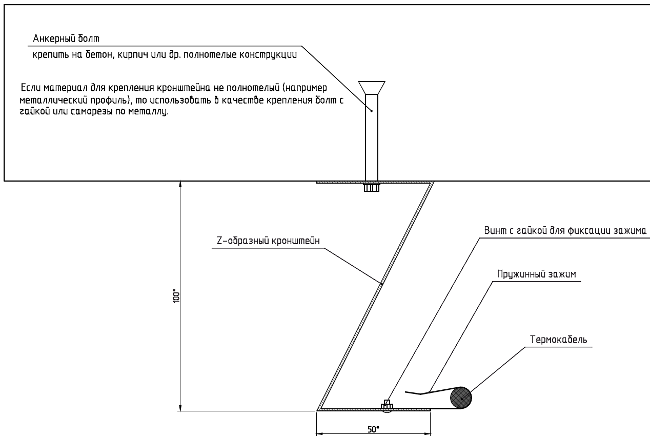
Рисунок 1. Чертеж МЭТ-01-01
