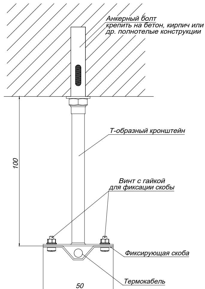
Рисунок 1. Чертеж МЭТ-01-02
