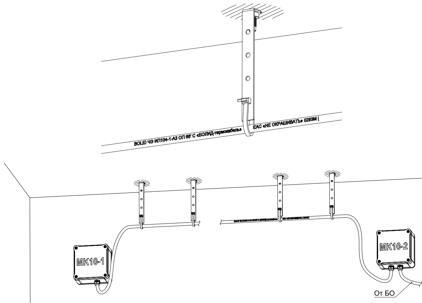
Рисунок 2. Пример размещения МЭТ-01-03
