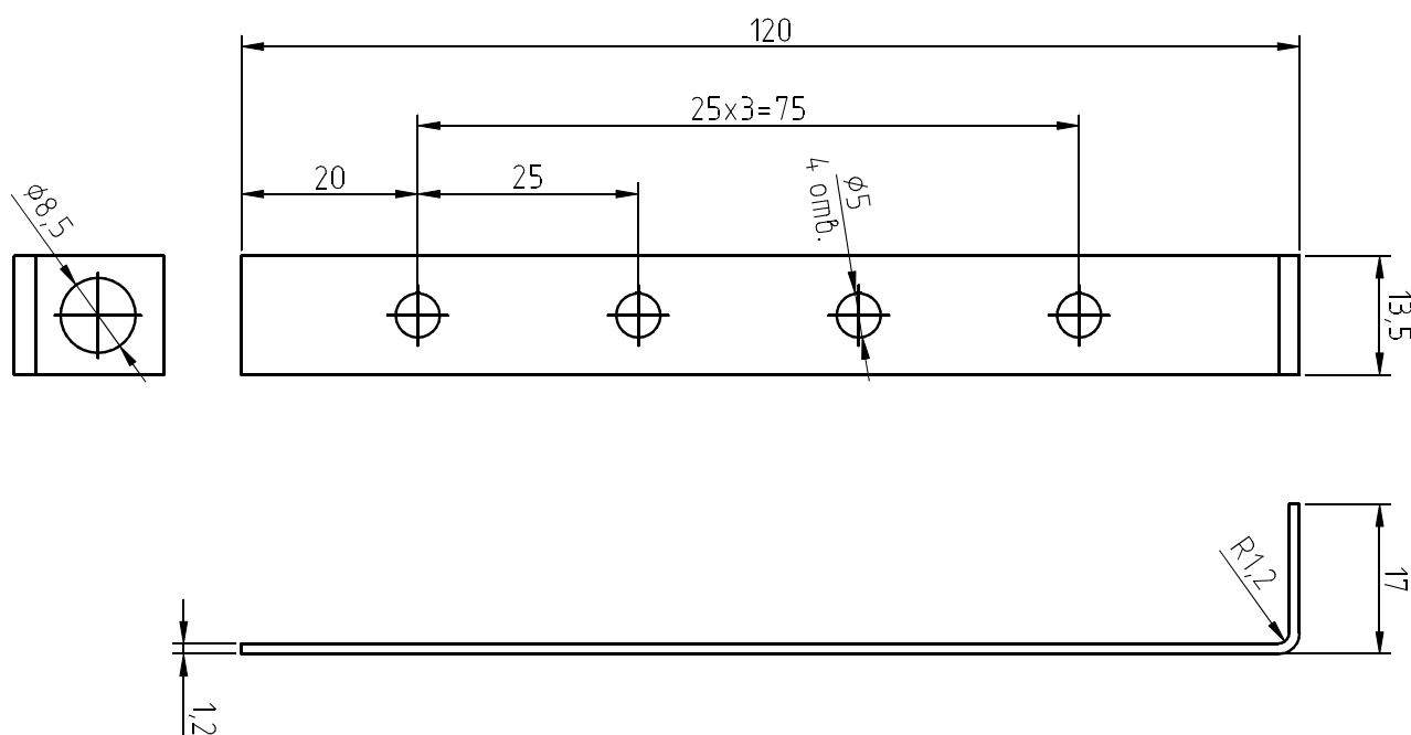
Рисунок 1. Чертеж МЭТ-01-03
