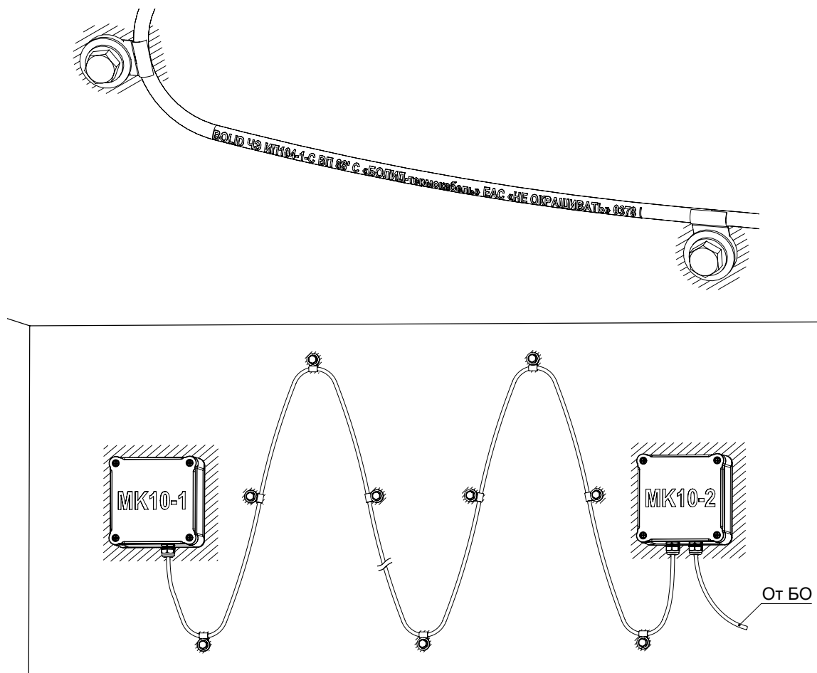
Рисунок 2. Пример размещения МЭТ-01-04
