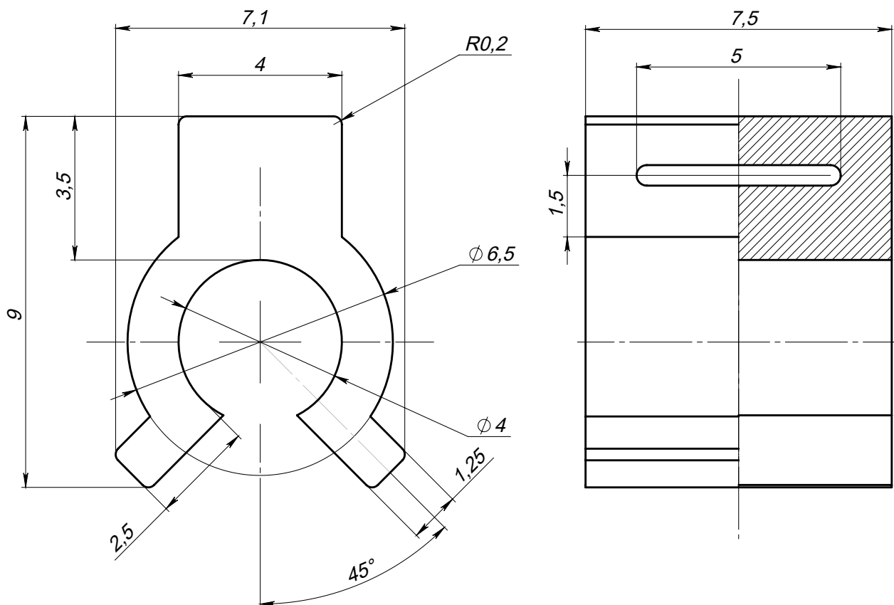
Рисунок 1. Чертёж МЭТ-02-01
