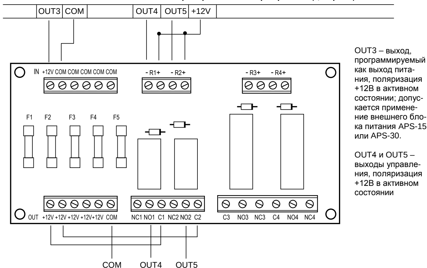
Рис. № 3. Пример применения модуля для замены выходов низкого тока (типа ОС) выходами высокого тока в приборе-сигнализаторе охранный (центральный) СА-6 плюс.
