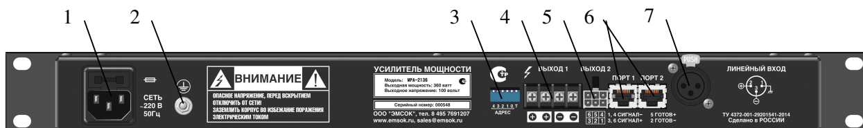
Рисунок 6.2. Задняя стенка коммутатора. 1 – Соединитель для подачи питания, 2 – клемма защитного заземления, 3 – переключатель задания адреса и включения терминатора, 4 – силовой выход, 5 – силовой выход с сигналом готовности, 6 – порты для подключения к БУС, 7 – аналоговый вход.
