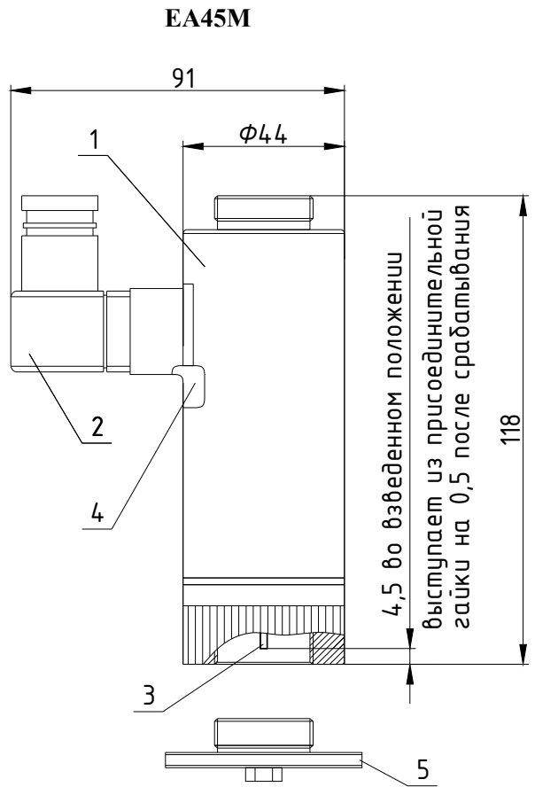
1 – Корпус; 2 – Электрический разъем; 3 – Пусковой шток; 4 – Гарантийная этикетка (при наличии); 5 – Пластиковая крышка.
