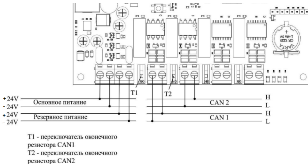
Рисунок 10 – Схема подключения интерфейса CAN и линии питания
