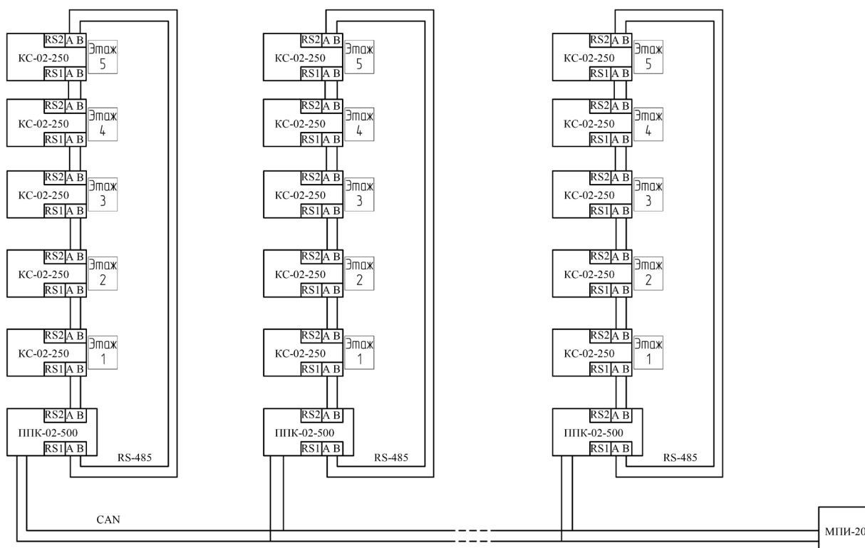
Рисунок 6 – Типовая схема подключения (для ППК-02-500)
