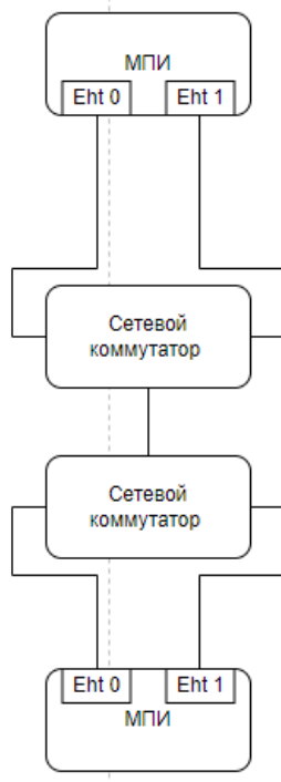
Рисунок 9 – Режим работы: два равнозначных интерфейса
