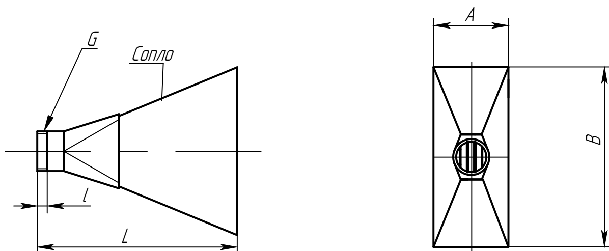
Общий вид насадков типов: НР-3.8, НР-6.12
