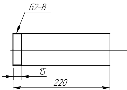
Общий вид насадка НРГ
