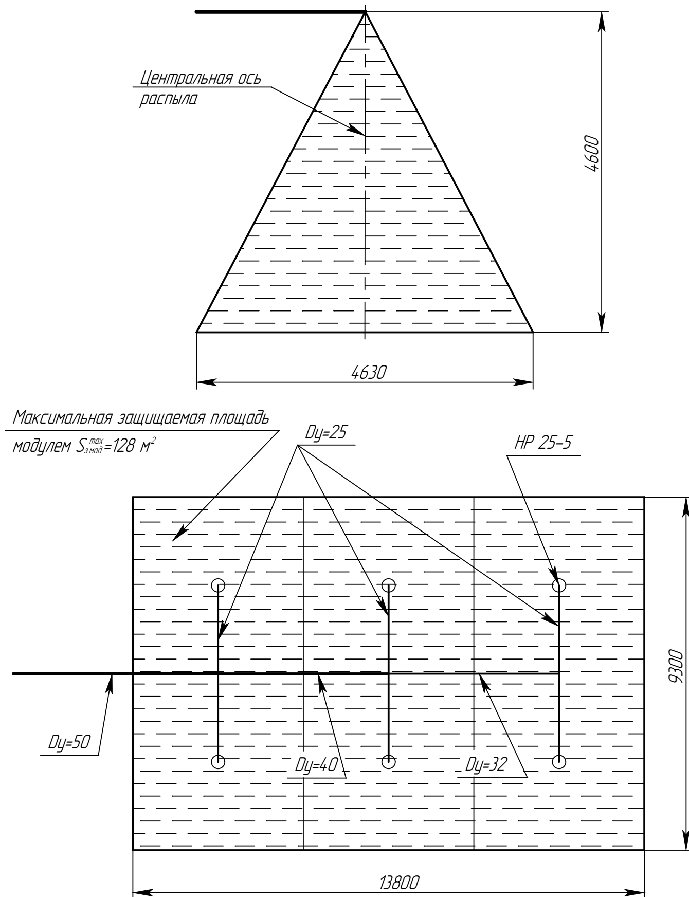
Рис. А12 Конфигурация максимальной защищаемой площади модуля с насадками HP 25-5 при их высоте размещения 4,6 м (вариант размещения 11)
