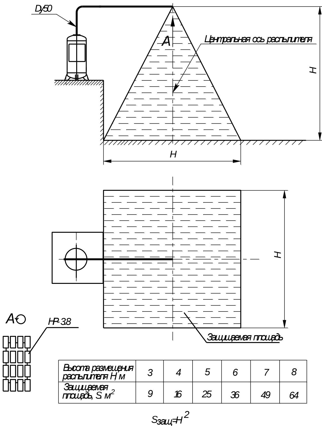
Рис. А7 - Конфигурация защищаемой площади модуля с насадком-распылителем НР-38 (варианта размещения б)
