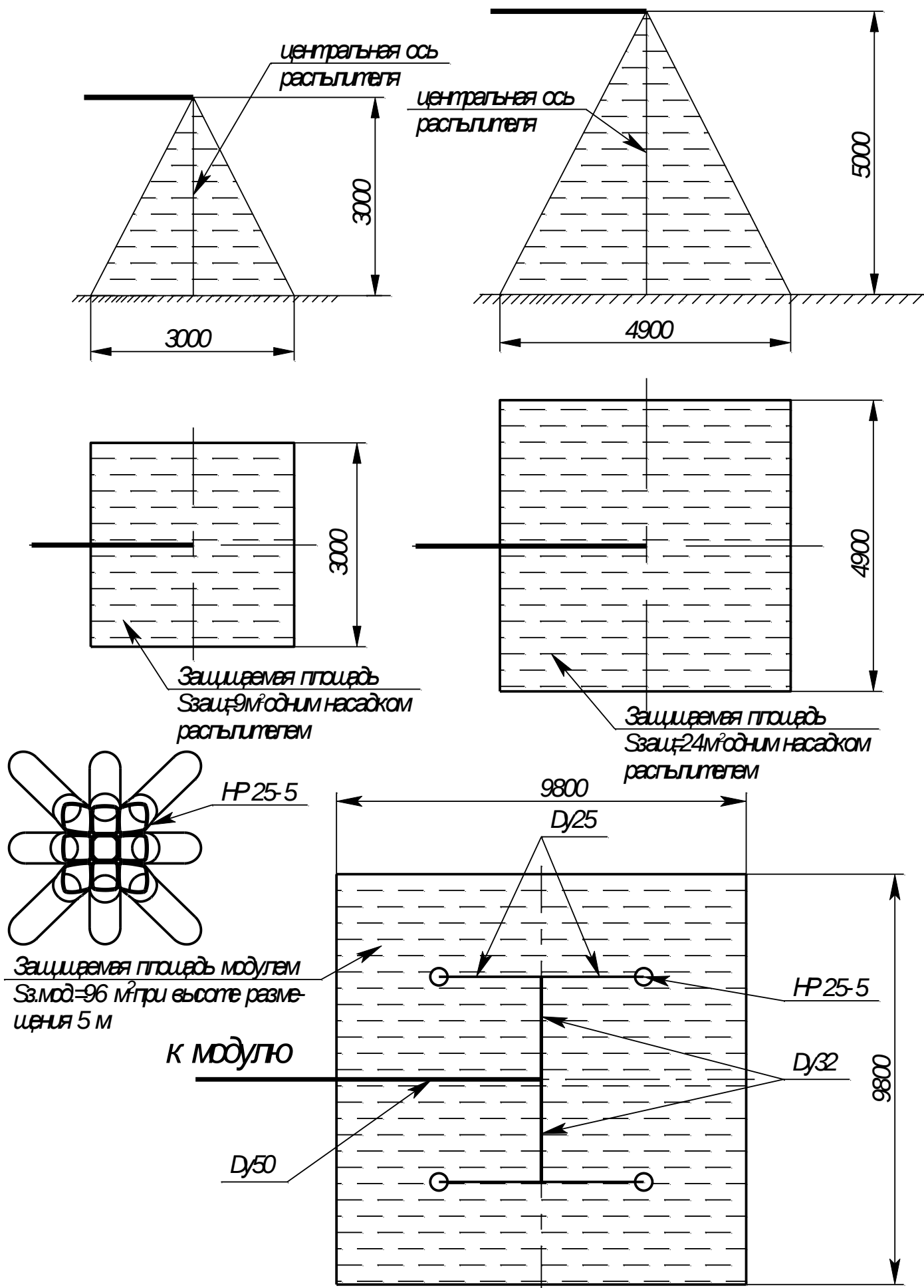
Рис. А11 - Конфигурация защищаемой площади модуля с насадком распылителя HP 25-5 при различной высоте размещения распылителя (варианта размещения 10)
