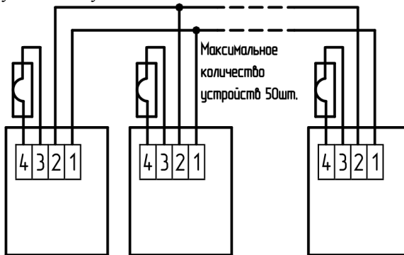
Рисунок 4 – Схема группового включения устройств
