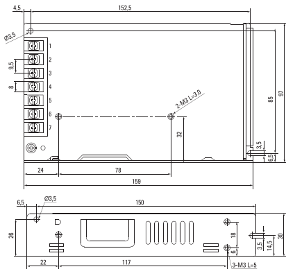
Рис 4. Габаритные размеры (MPS-150W-24)
