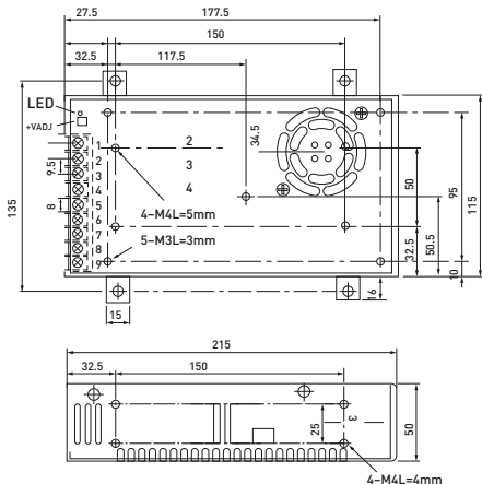
Рис 6. Габаритные размеры (MPS-500W-12)
