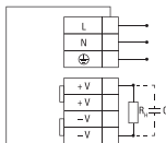
Рис 8. Схема подключения (MPS-100W-12, MPS-150W-12)
