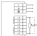
Рис 9. Схема подключения (MPS-200W-12, MPS-350W-12, MPS-500W-12)
