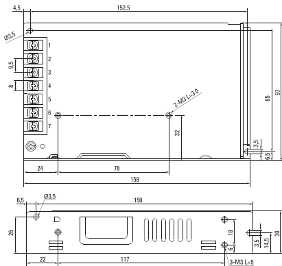
Рис 4. Габаритные размеры (MPS-150W-12)
