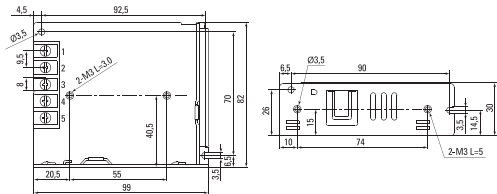
Рис 1. Габаритные размеры (MPS-35W-12, MPS-50W-12)
