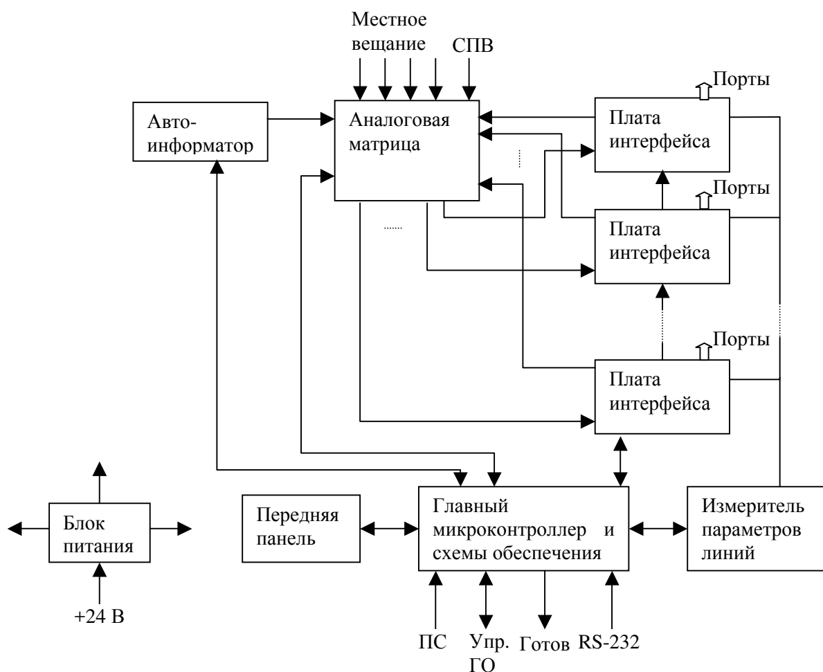
Рисунок 6.4. Структурная схема БУС.
