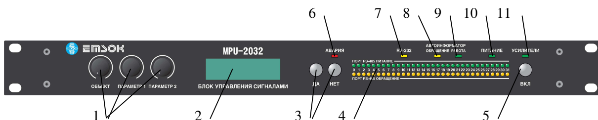
Рисунок 6.1. Передняя панель БУС. 1 – Поворотные переключатели, 2 – ЖКД, 3 – кнопки управления «Да» и «Нет», 4 – индикаторы режимов работы портов, 5 – кнопка управления режимом питания «Вкл», 6 – индикатор неисправности СОУЭ, 7 – индикатор обращения по порту RS232, 8 – индикатор обращения к автоинформатору, 9 – индикатор обращения к памяти автоинформатора, 10 – индикатор подачи питания на БУС, 11 – индикатор режима питания.
