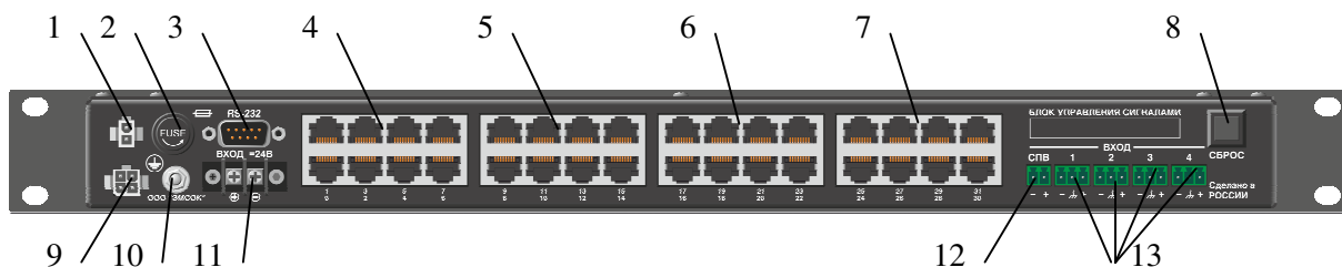
Рисунок 6.2. Задняя стенка БУС. 1 – Вывод сигнала исправности, 2 – держатель предохранителя, 3 – порт RS-232, 4 – порты 1-8, 5 – порты 9-16, 6 – порты 17-24, 7 – порты 25-32, 8 – кнопка перезагрузки, 9 – интерфейс управления СПВ, 10 – клемма заземления, 11 – клеммник подачи питания, 12 – вход СПВ, 13 – входы МВ.
