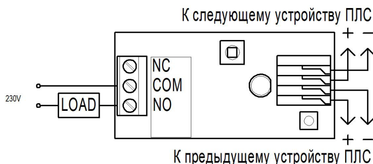
Рисунок 5 – Схема подключения
