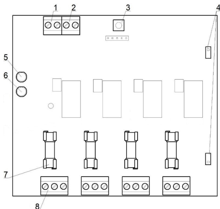
Рисунок 2 – Внутреннее устройство модуля
