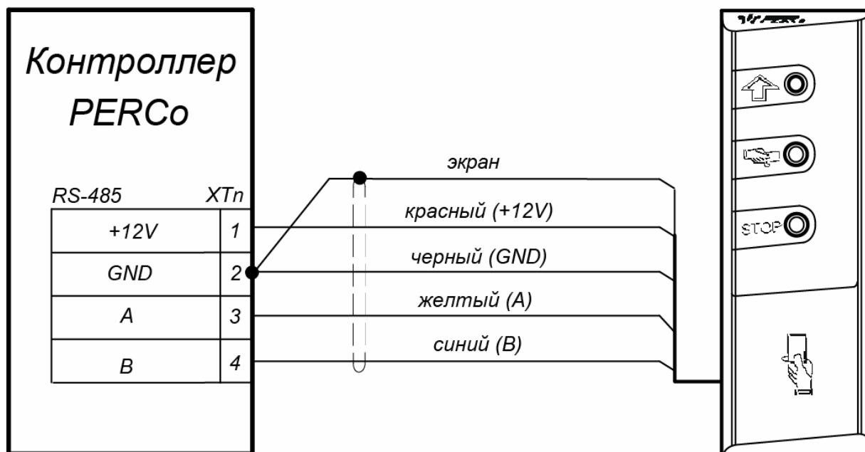
Рисунок 3. Схема подключения считывателя к контроллеру PERCo
