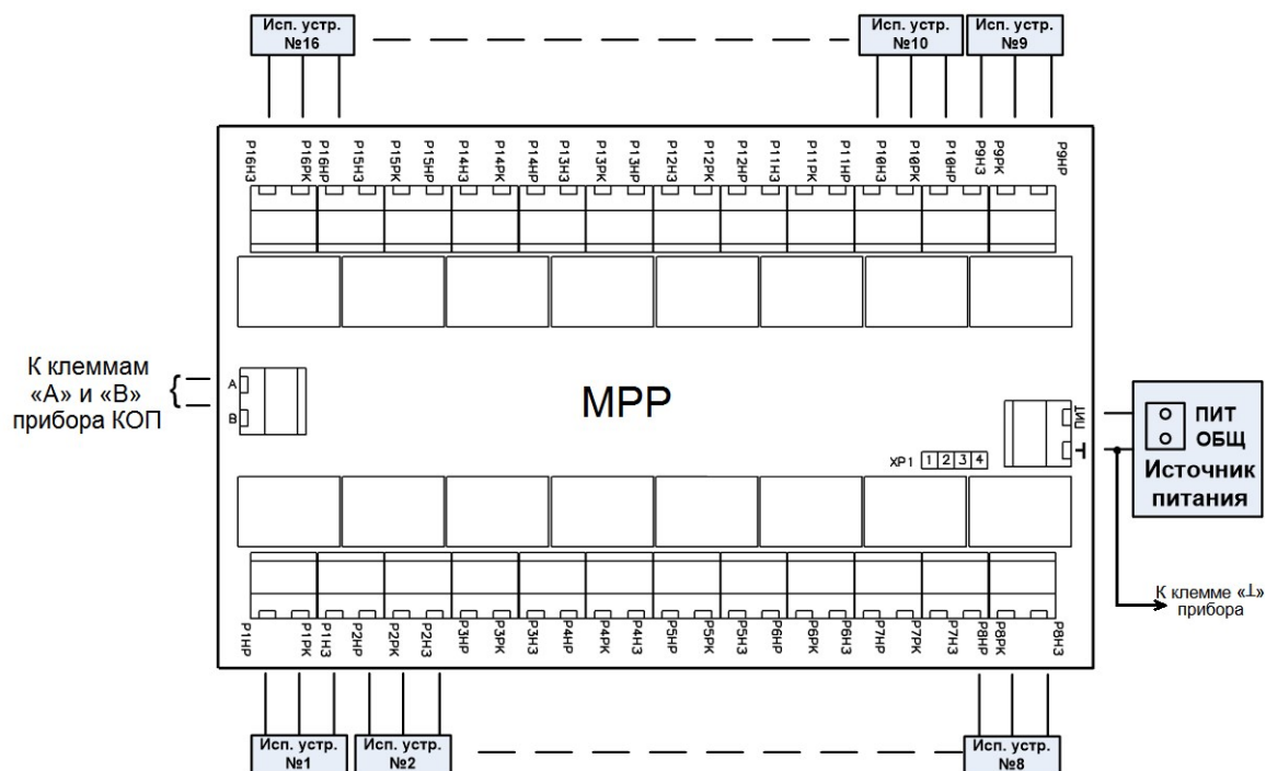
Рисунок 1. Схема подключения
