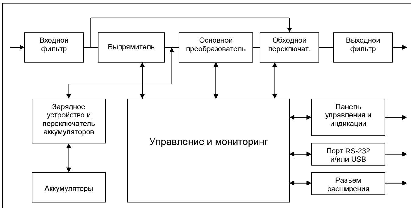
Рис. 6. Блок-схема ИБП
