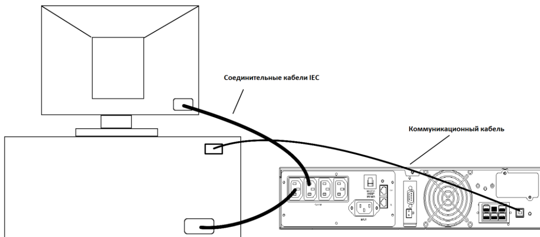
Рис. 4. Пример подключения устройств Plug&Play
