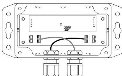
Вариант подключения проводников повышенной жесткости
