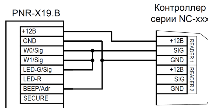
Рисунок 6. Подключение считывателя по интерфейсу Parsec, адрес 0 (наружный)
