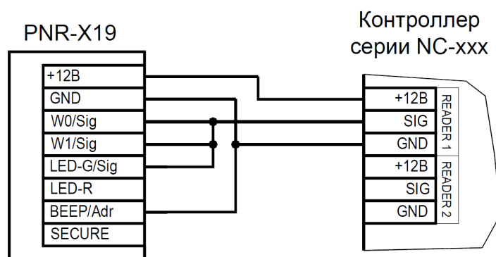
Рисунок 5. Подключение считывателя по интерфейсу Parsec, адрес 1 (внутренний)
