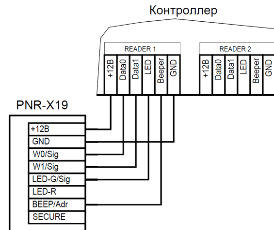
Рисунок 4. Подключение считывателя по интерфейсу
