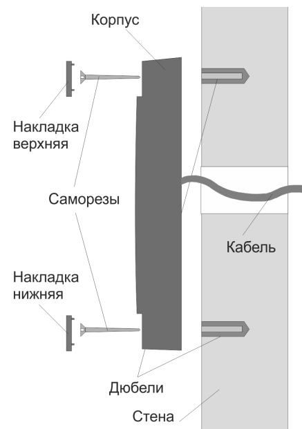
Рисунок 2. Крепление считывателя
