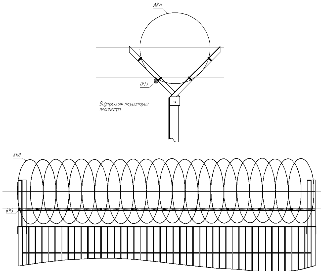
Рисунок 2.8 – Установка ВЧЭ на объемный АКЛ
