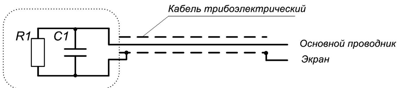
Рисунок 2.5 – Конструкция ВЧЭ
