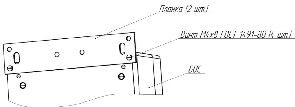
Рисунок 2.4 – Крепление планки к БОС
