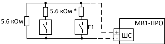
Рис.5. Подключение к ШС пожарных извещателей с нормально разомкнутой выходной цепью
