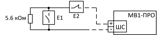
Рис.3. Подключение к ШС извещателей технологической сигнализации
