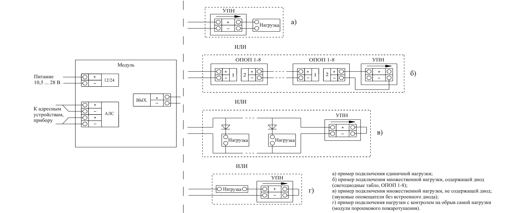
Схема подключения модуля
