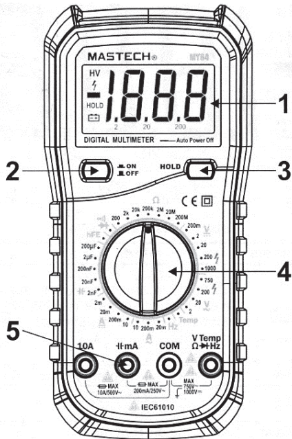
Рисунок 1. Схема мультиметра
