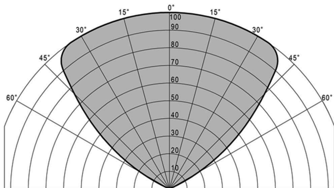
Рисунок 5 - Зависимость дальности обнаружения очага пламени от его углового положения в поле зрения извещателя в процентах от максимального значения
