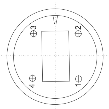
Схема расположения контактов основания.
