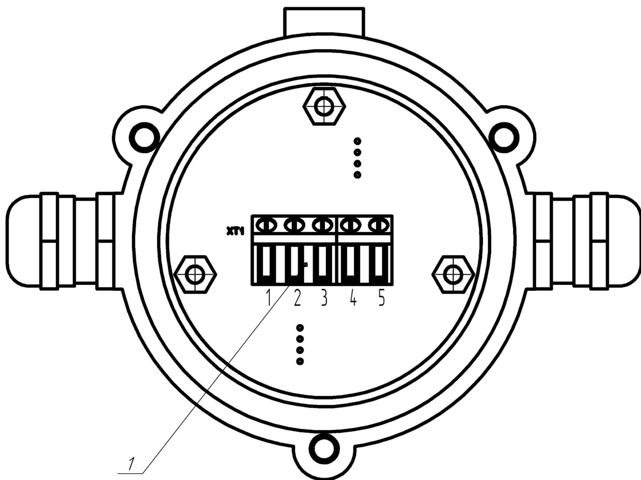
Рисунок 2 - Внутренняя часть извещателя.
