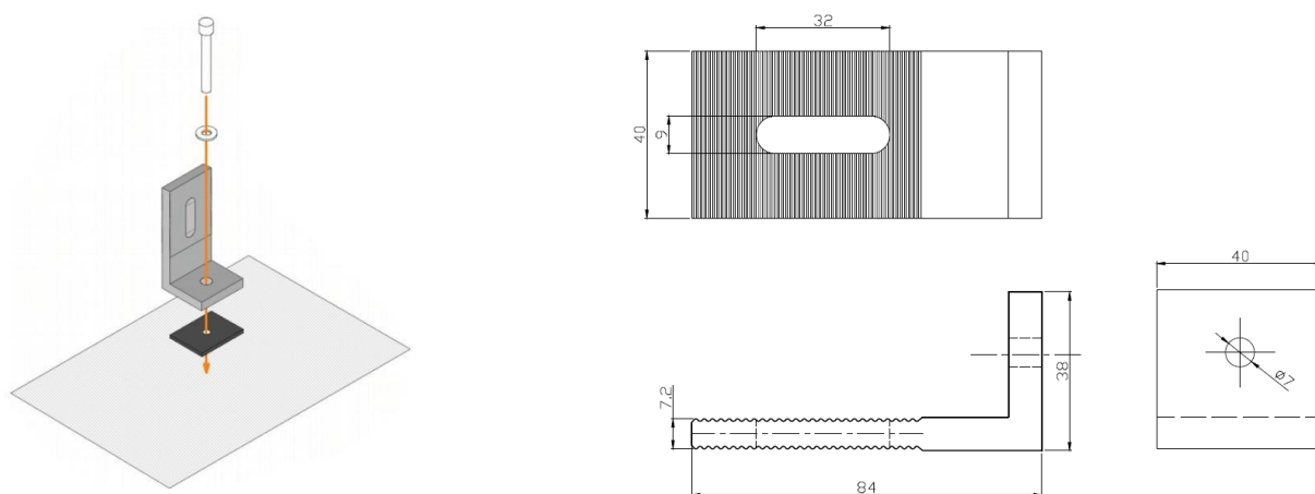
Рисунок 17. L-образное крепление универсальное.
