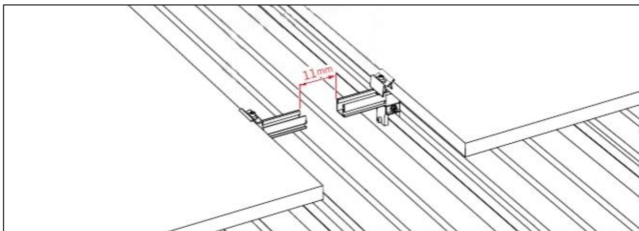
Рисунок 20. Температурный зазор между металлическими профилями.
