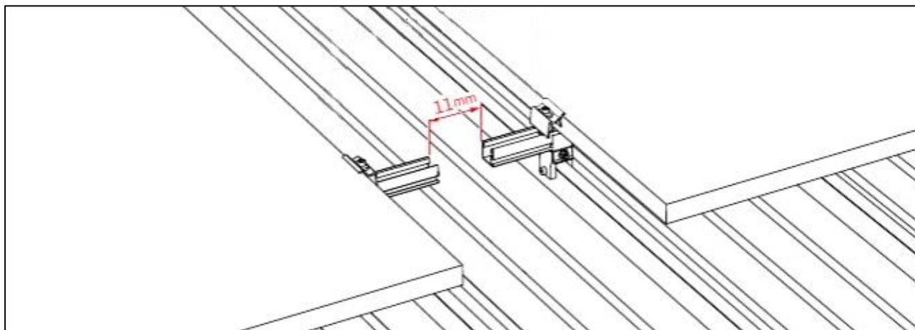
Рисунок 11. Температурный зазор между металлическими профилями.
