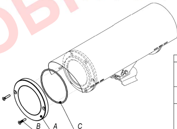
Рис.1 Установка НС-8 на термокожух ТГБ-8Г(Р) Ех
