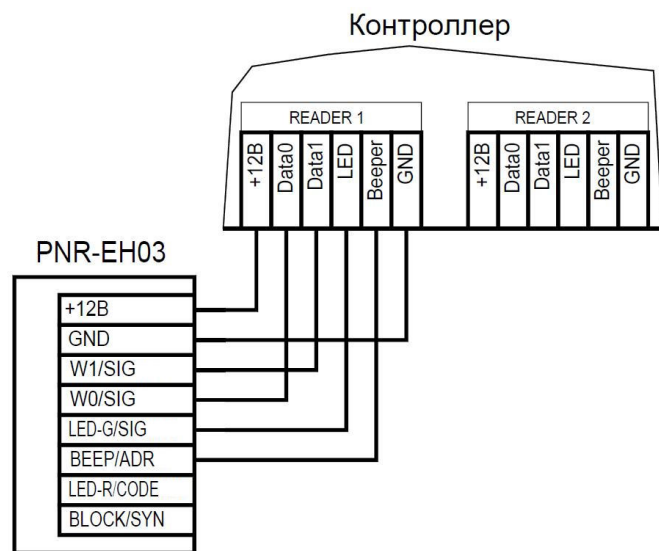
Рисунок 7. Подключение считывателя по интерфейсу Wiegand
