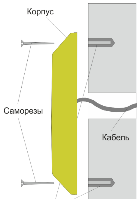
Рисунок 2. Крепление считывателя
